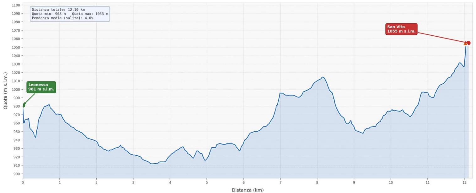
Profilo Altimetrico — SI O16 | Leonessa > San Vito
