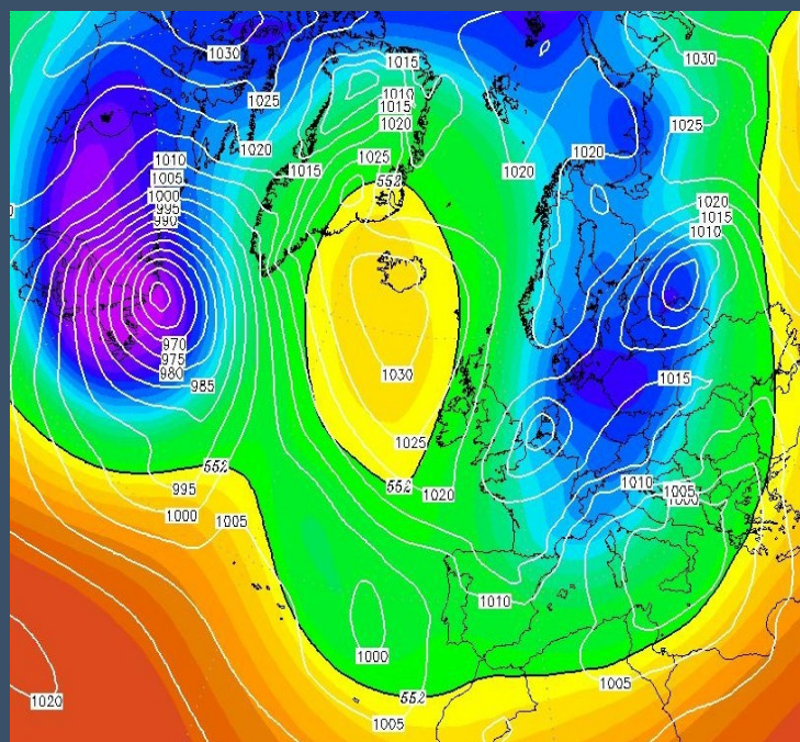
ondata di gelo del gennaio 1985. archivio wetterzentrale
